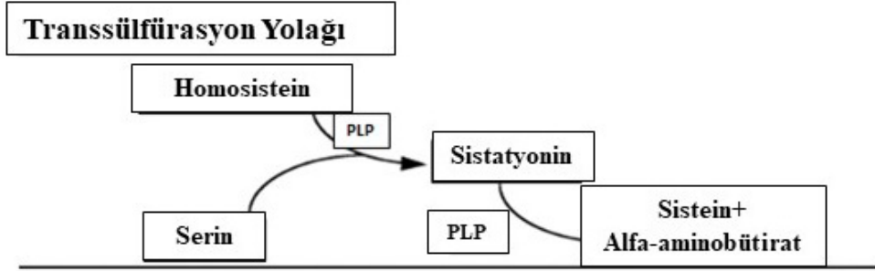
Şekil 4. Homosistein Transsülfürasyon Yolu (PLP: Piridoksal fosfat) (Lynn B. Bailey ve Gregory, 1999)
